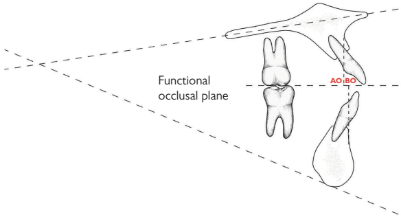
Fig. 4.8 Wits analysis.
